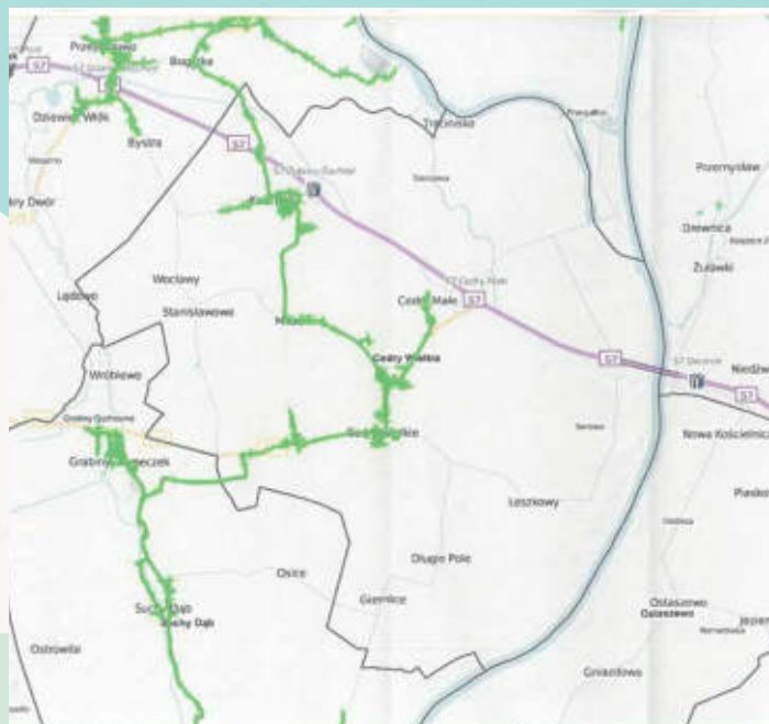
Na zdjęciu: Mapa przedstawiająca rozproszony układ trasy rurociągu.
